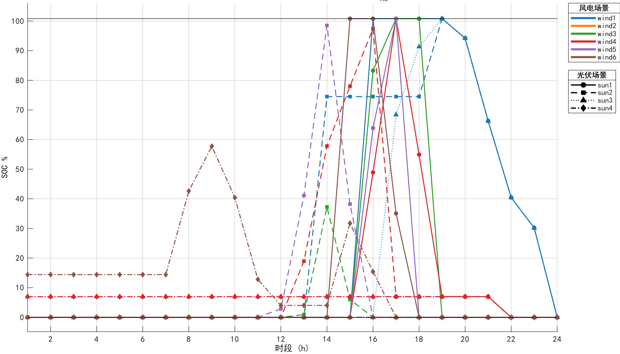
24 场景下电池储能 SOC 时序 (颜色=风电场景, 线型=光伏场景, E_{cap}=10.08 \text{ MW} \cdot \text{h} )
